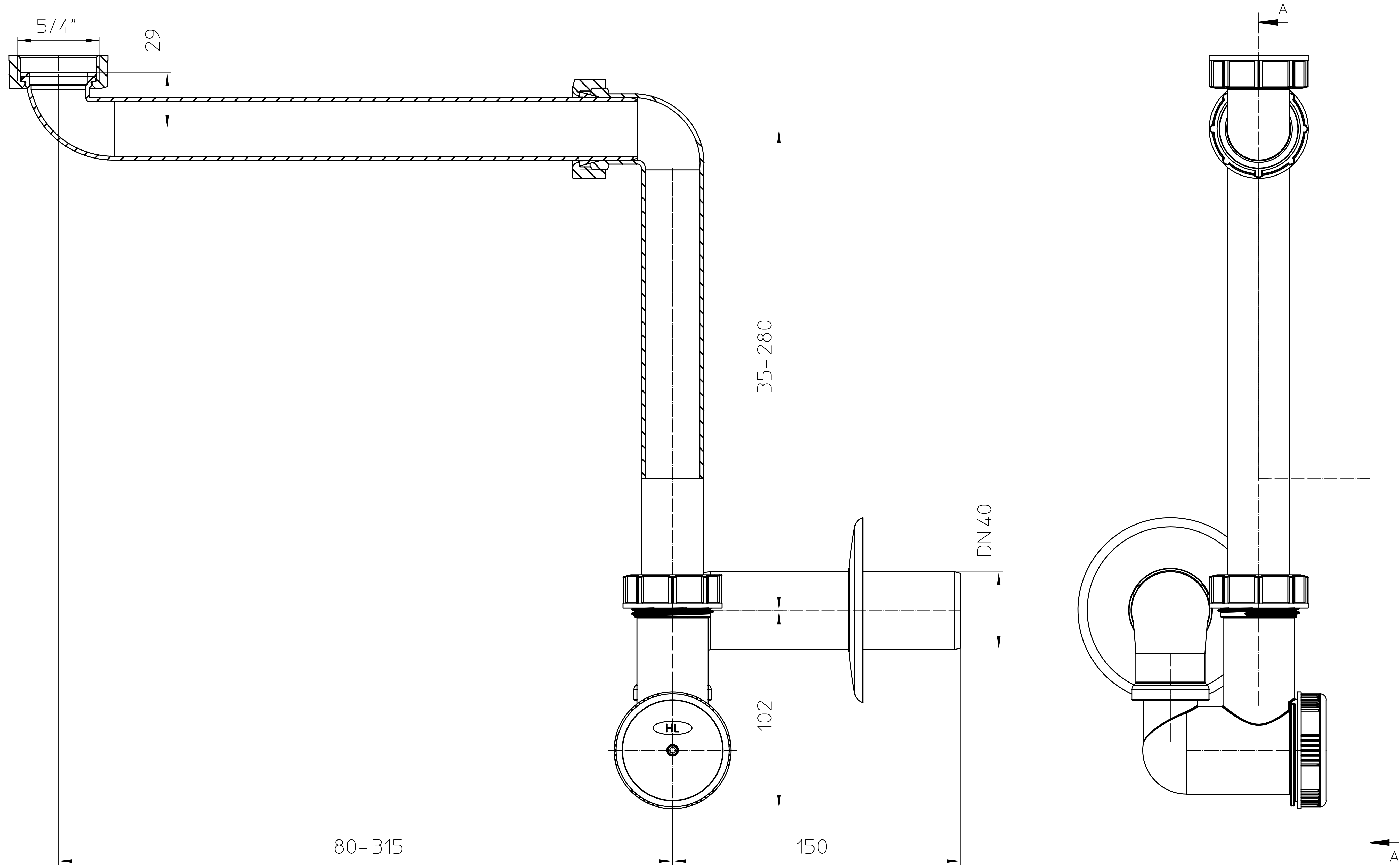
Schnitt A-A
