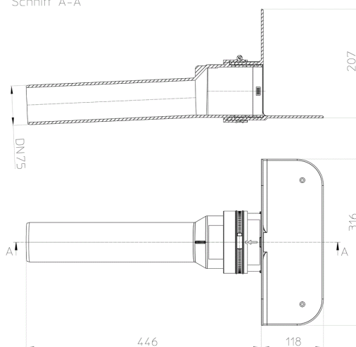
Schnitt A-A
