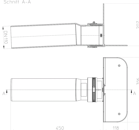
Schnitt A-A
